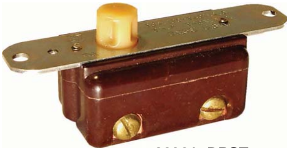
82321 DPST OFF - MOM. ON 20 amp. 125 volt
