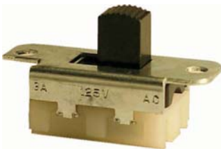
18-387 SPST OFF - MOM. ON S-60-A ON - OFF 4 amp. 125 volt
