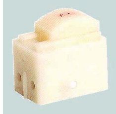
FU202 DPDT 4A 250V
