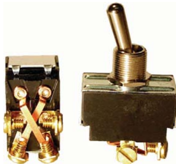
1276R DPDT ON - OFF - ON 15 amp. 125 volt
