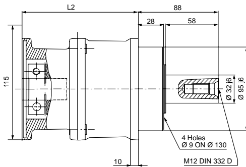
GBSM90-MNT115-XX
